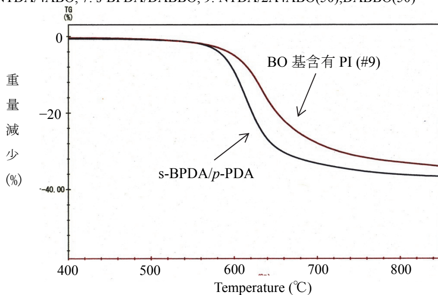
図4 BO基含有PIフィルム(#9)のTGA曲線
